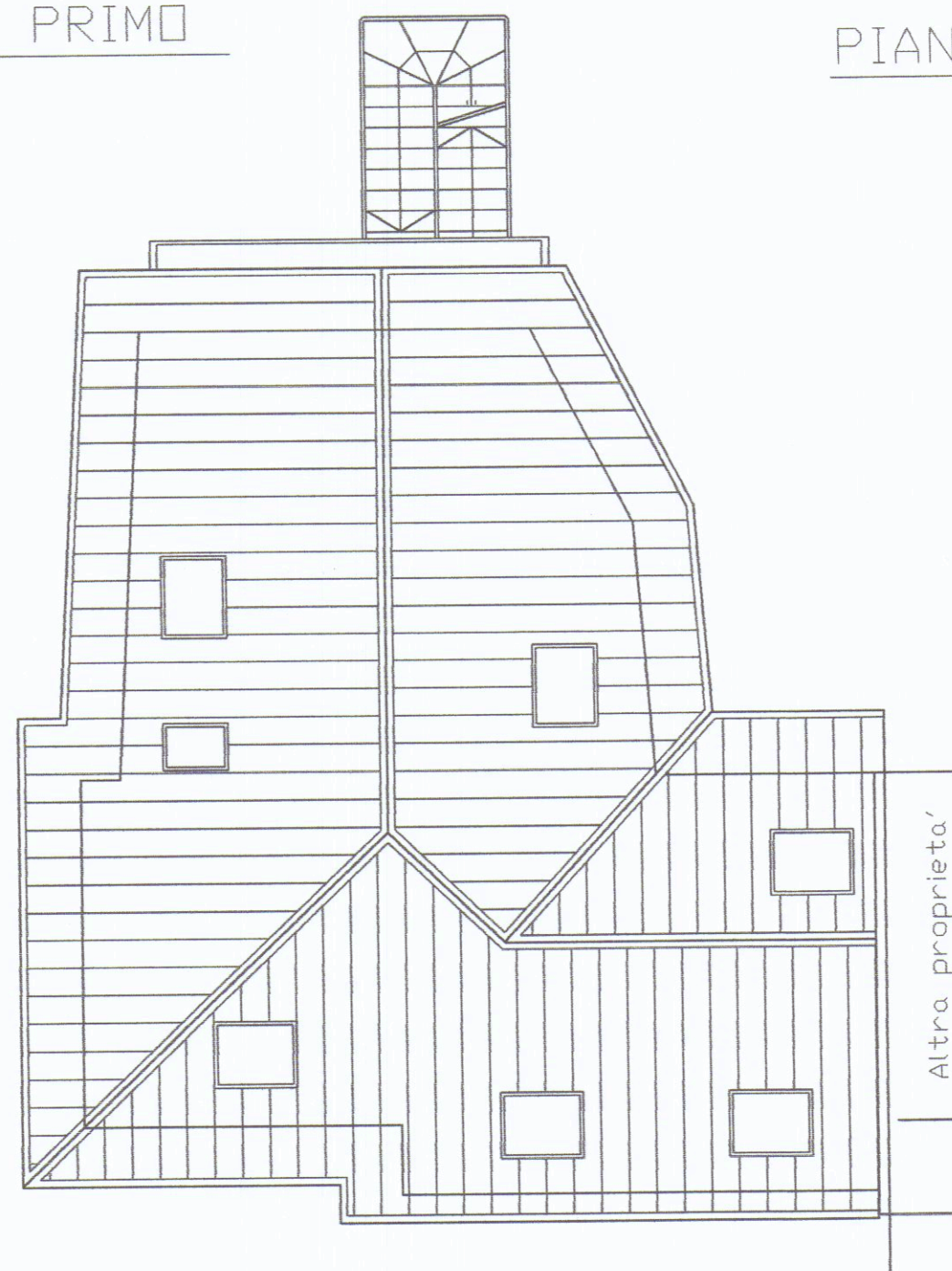
PIANTA COPERTURA
