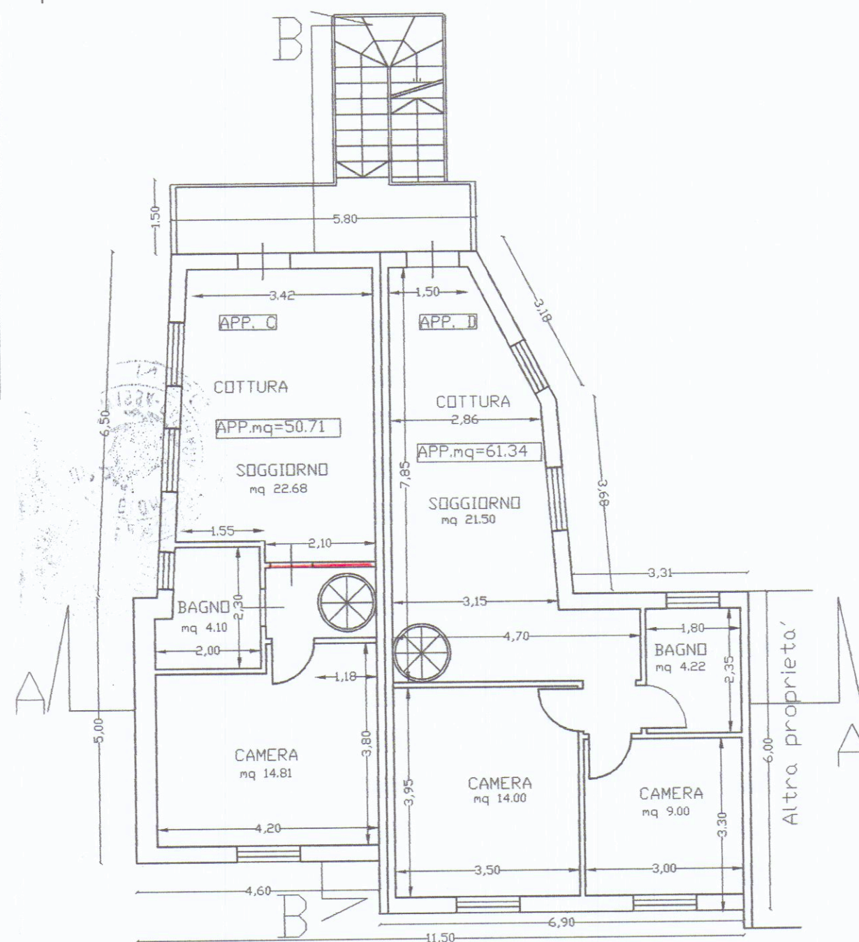
PIANO PRIMO
