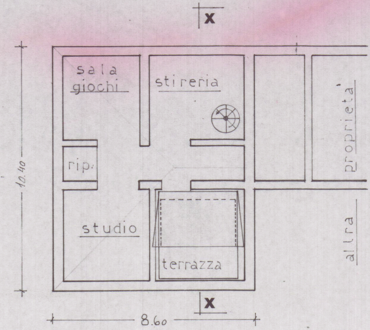
PIANTA SOTTOTETTO
