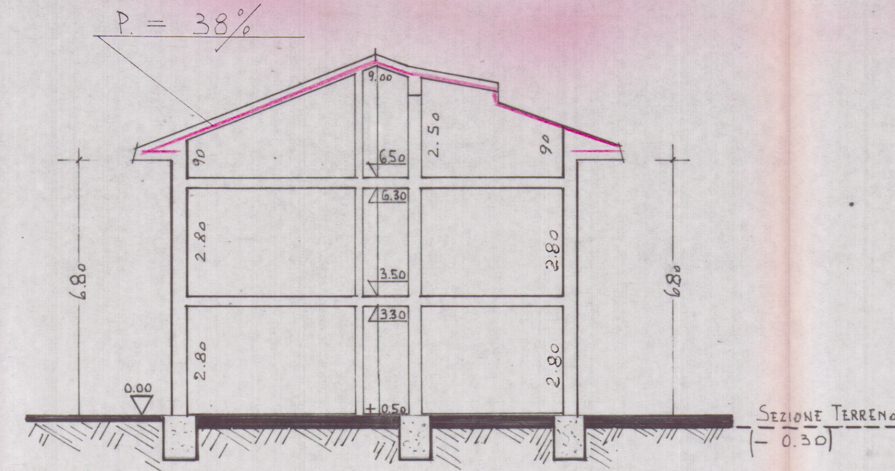
SEZIONE X-X
