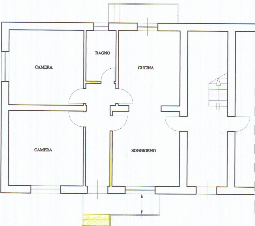
PIANTA ESISTENTE
