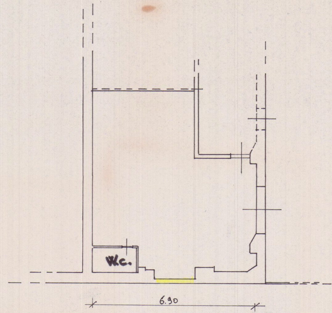
PIANTA ATTUALE
