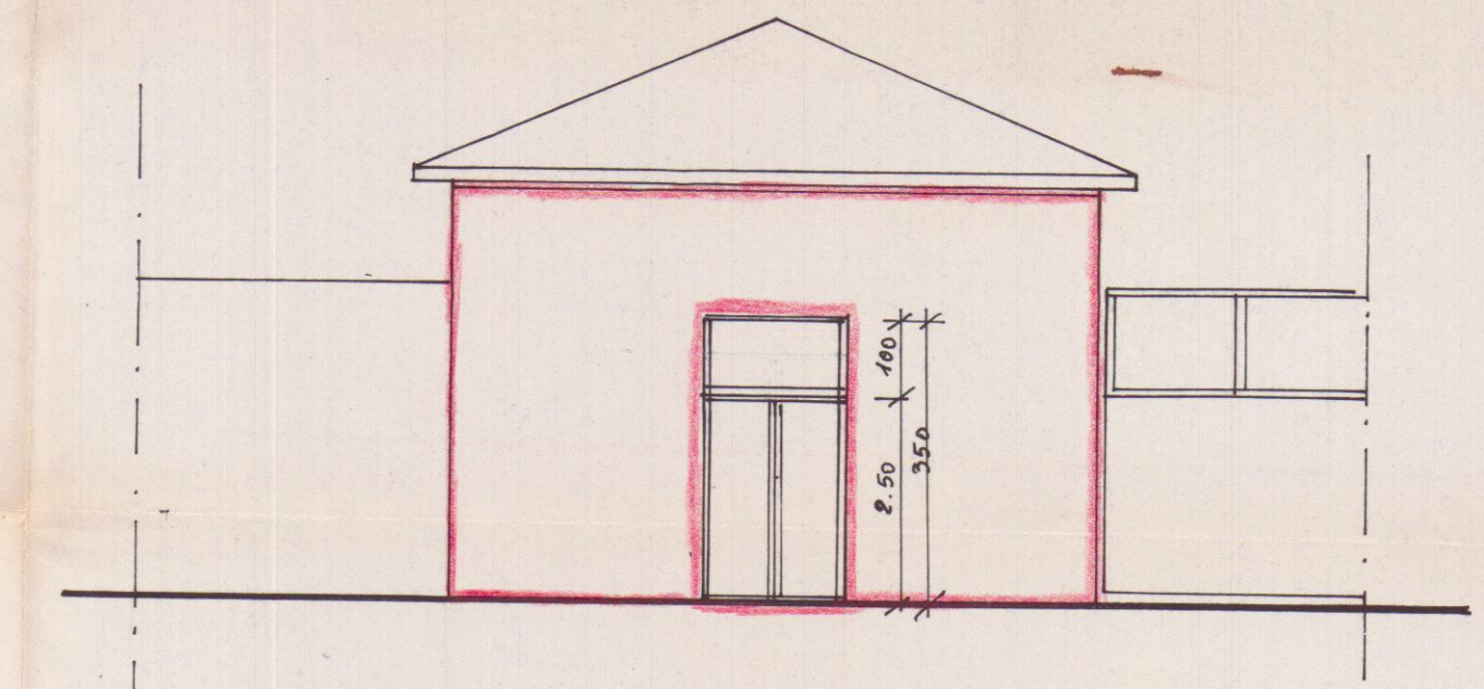
PROSPETTO MODIFICATO
