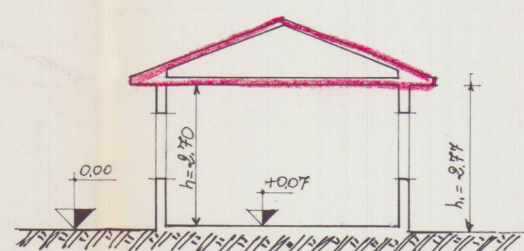
SEZIONE "A-A"
