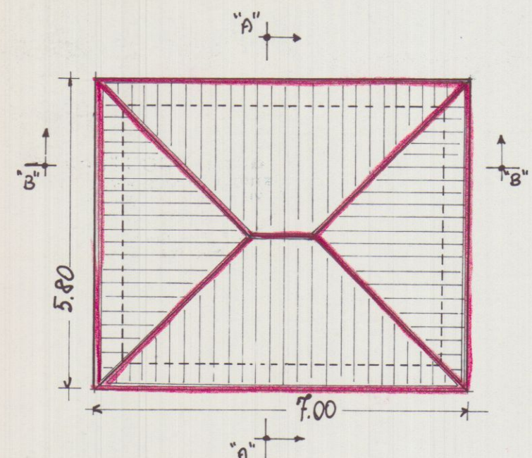
PIANTA COPERTURA
