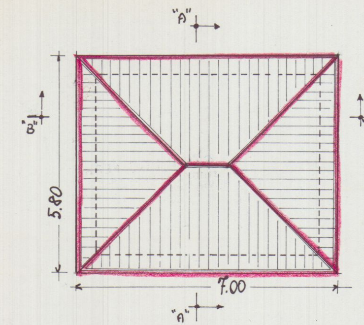
PIANTA COPERTURA
