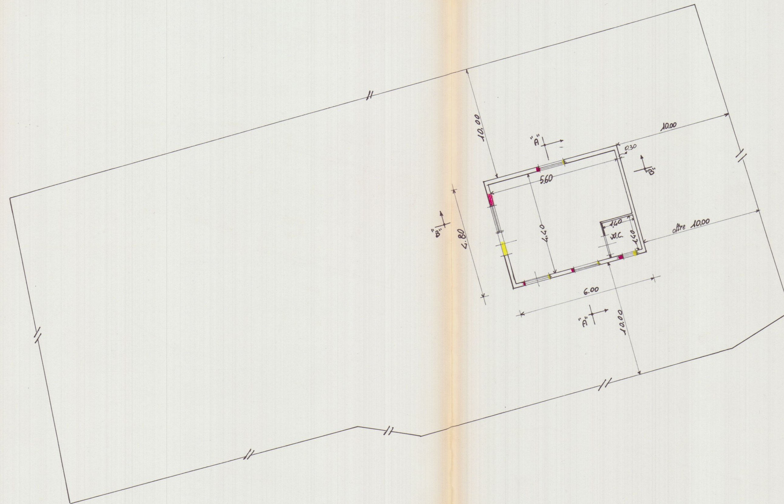
PLANIMETRIA GENERALE 1:100
