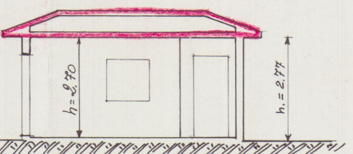
SEZIONE "B-B"
