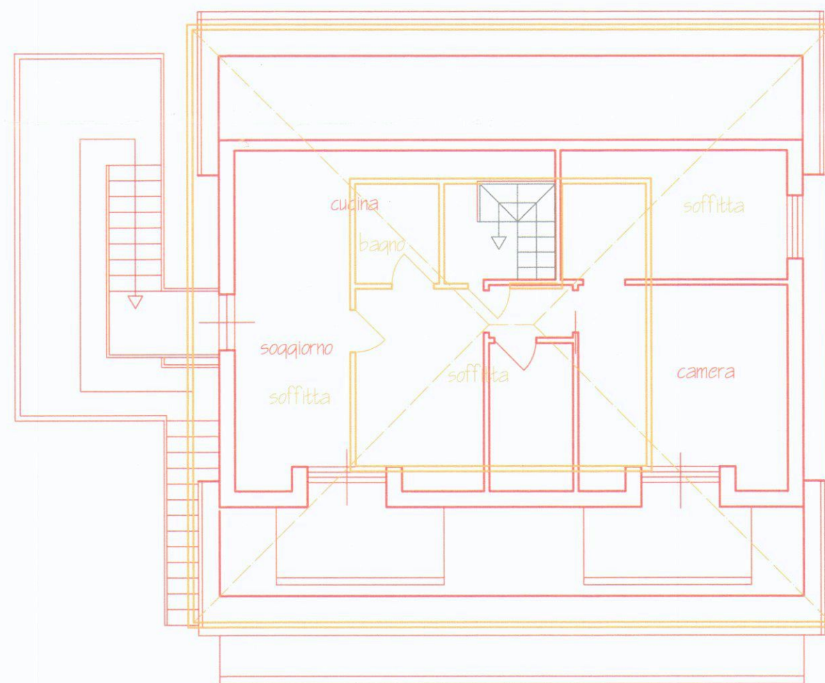
Piano Sottotetto
