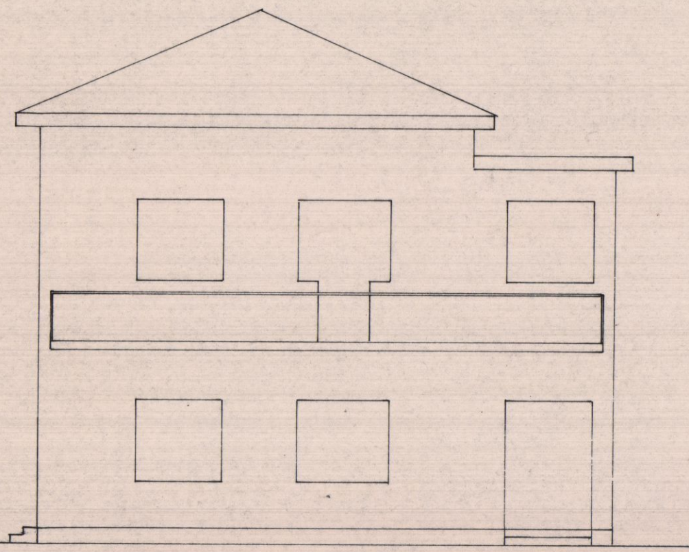
PROSPETTO EST
