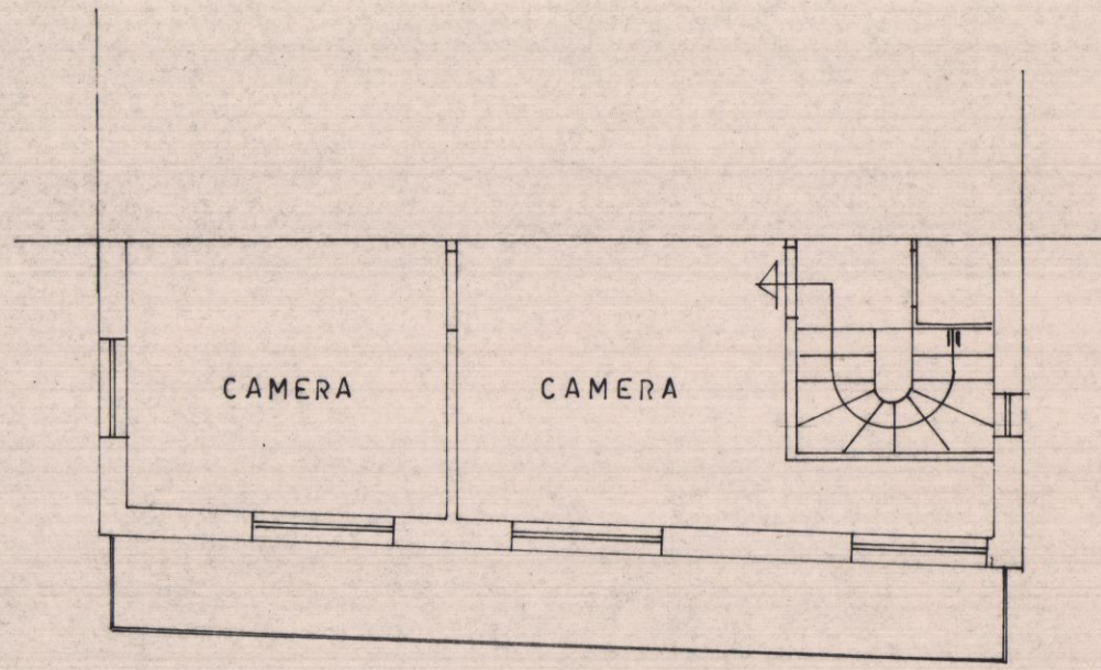
PIANO PRIMO
