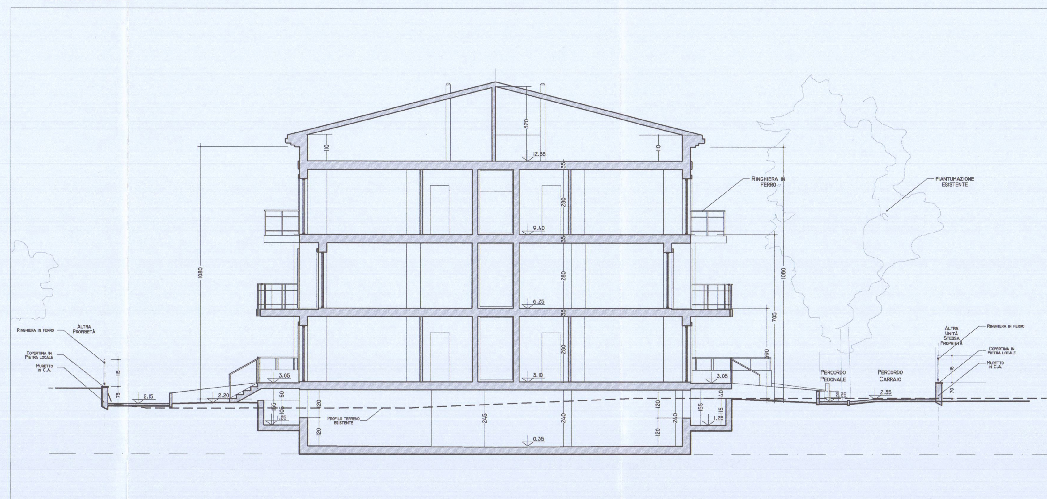
SEZIONE B-B
