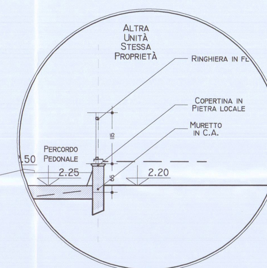
PARTICOLARE RECINZIONE SCALA 1:50
