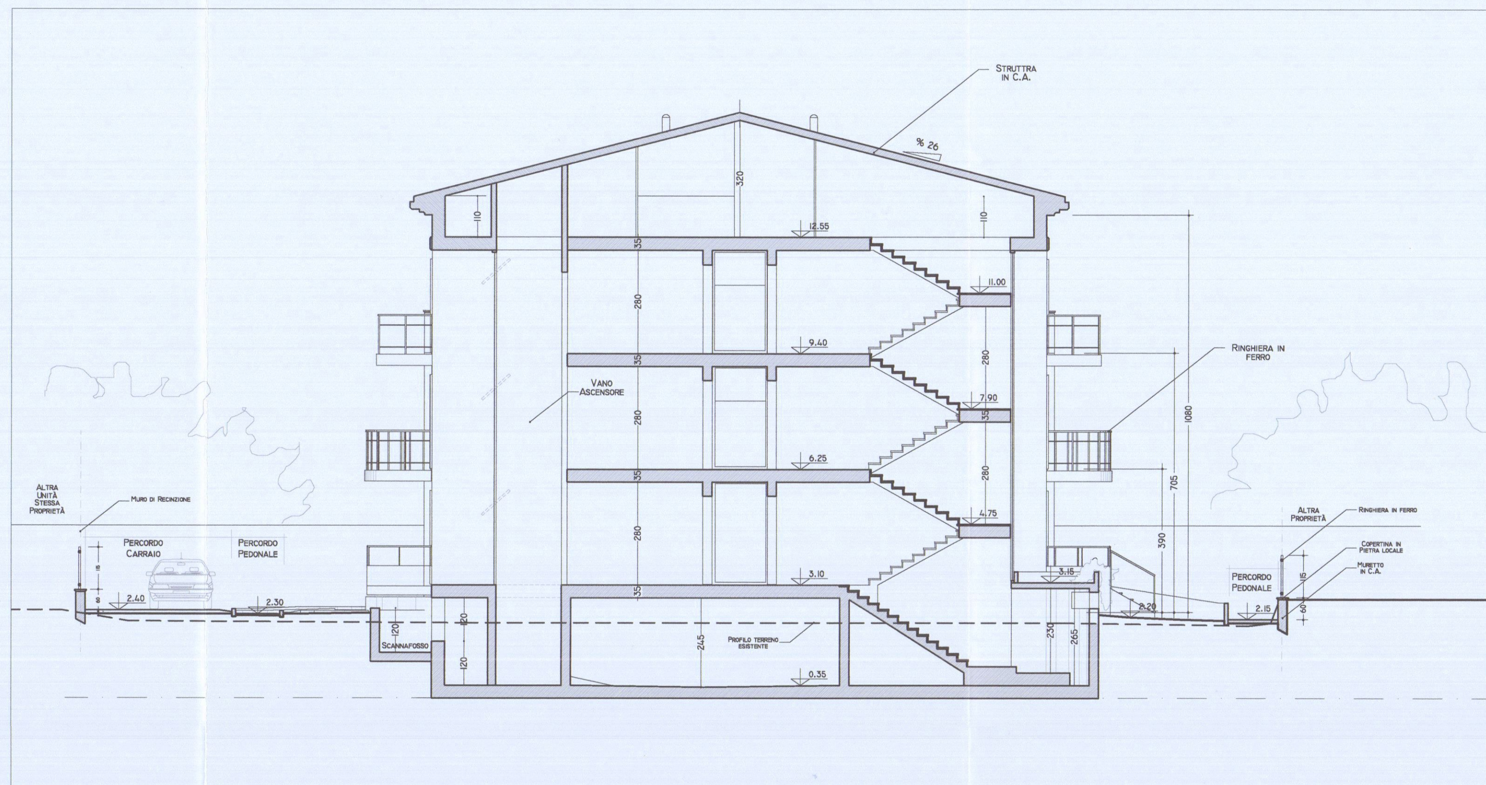
SEZIONE A-A
