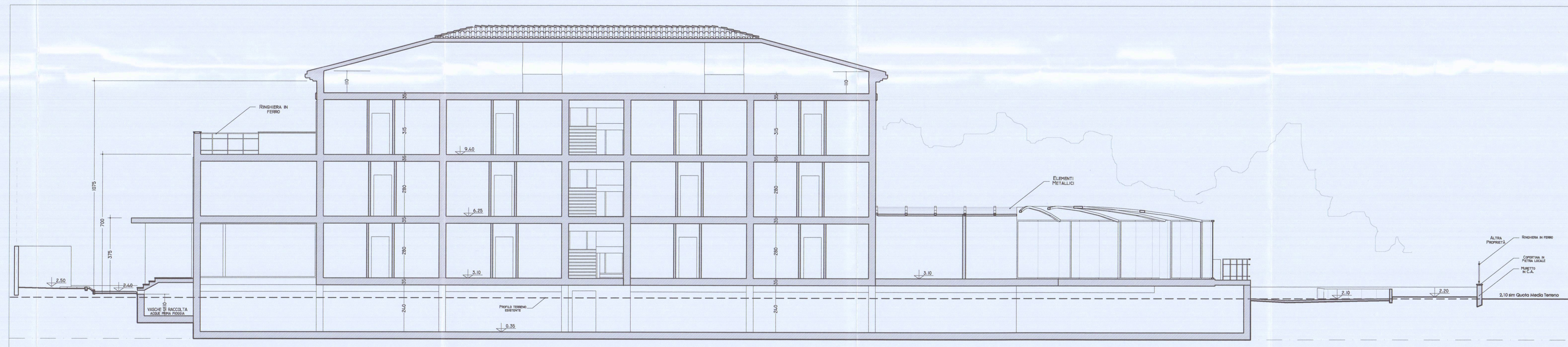
SEZIONE C-C
