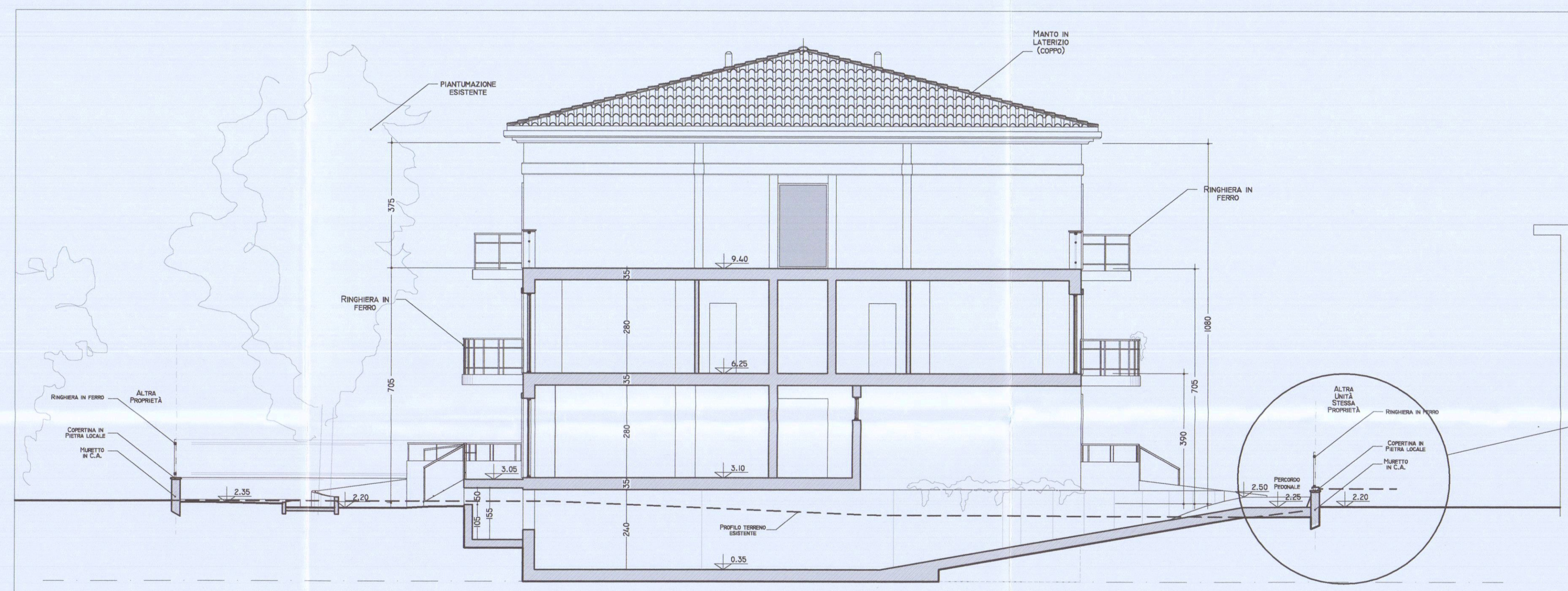
SEZIONE D-D
