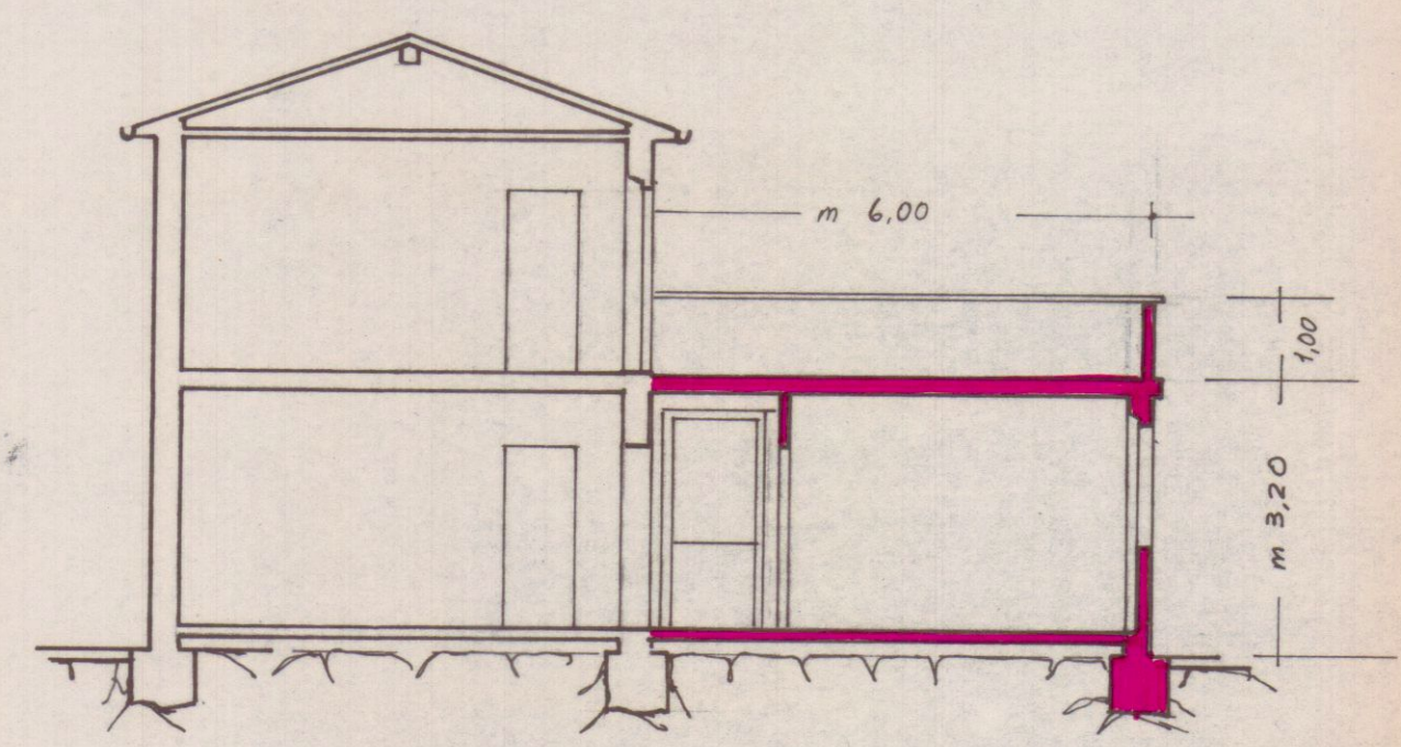
SEZIONE
