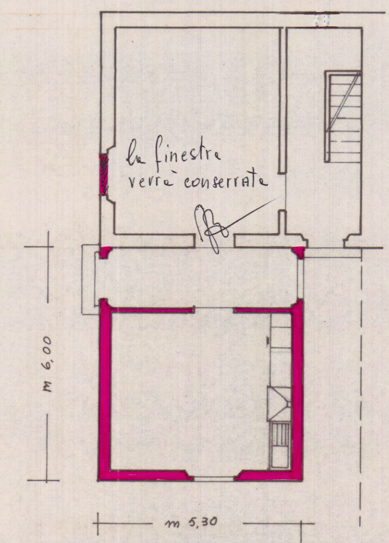
PIANTA AMPLIAMENTO ED ESISTENTE PIANO TERRENO
