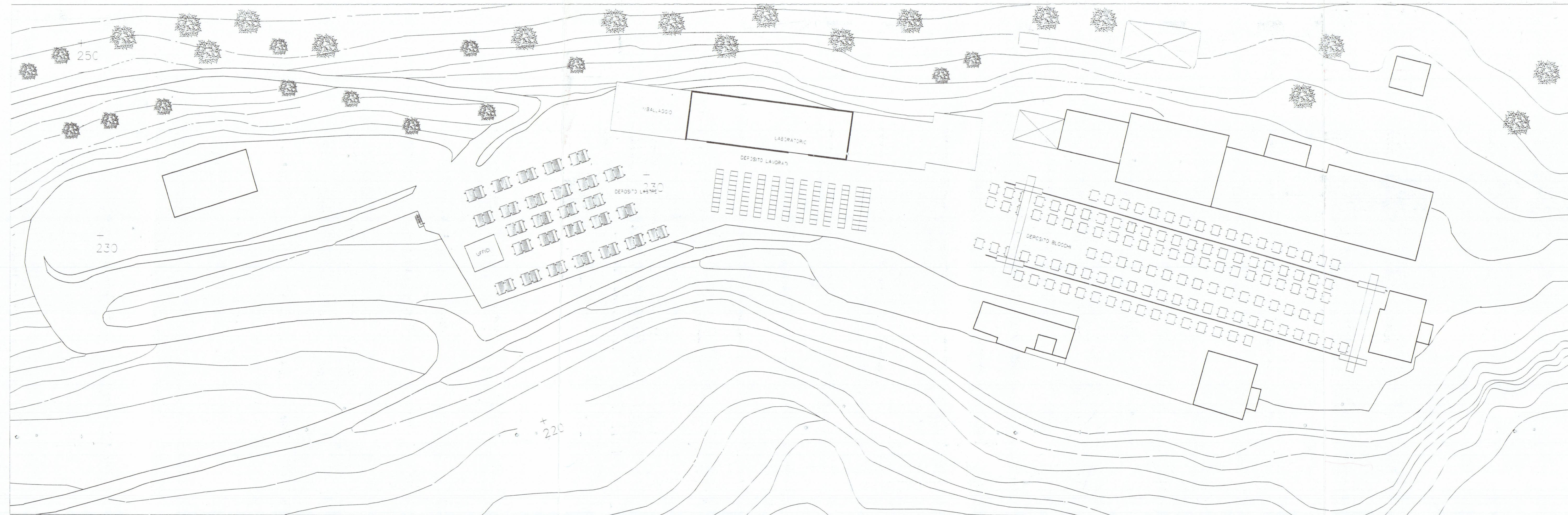
Planimetria generale compendio industriale La Facciata – planimetria scala 1/500
