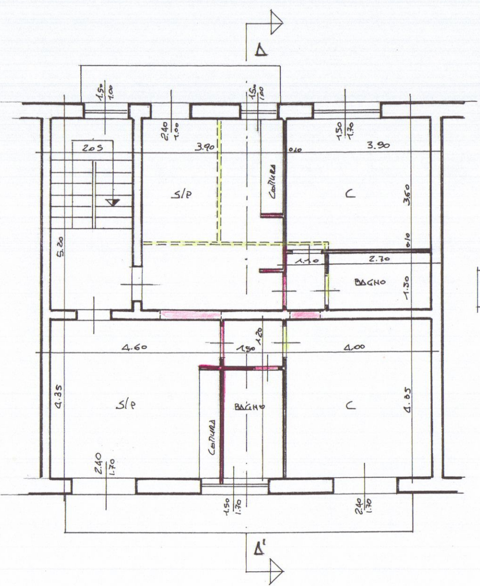
PIANTA P. PRIMO
