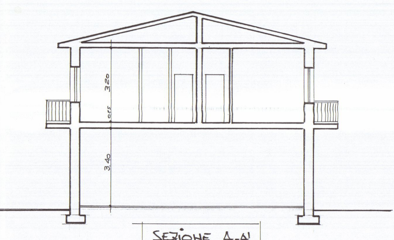
SEZIONE A-A'
