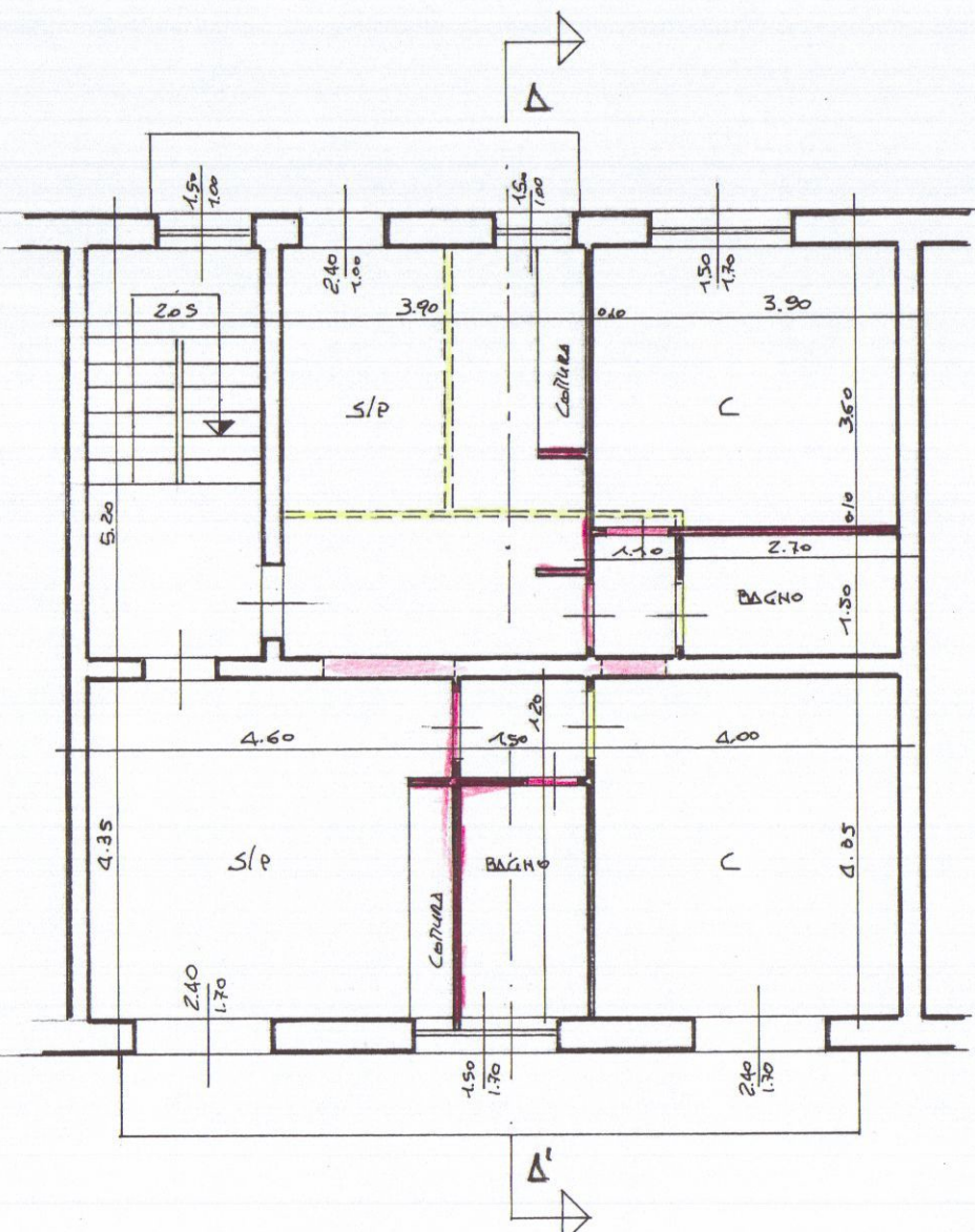
PIANTA P. PRIMO
