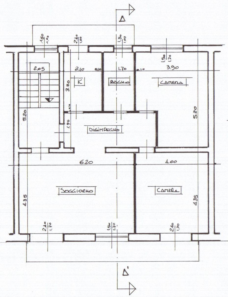
PIANTA P. PRIMO
