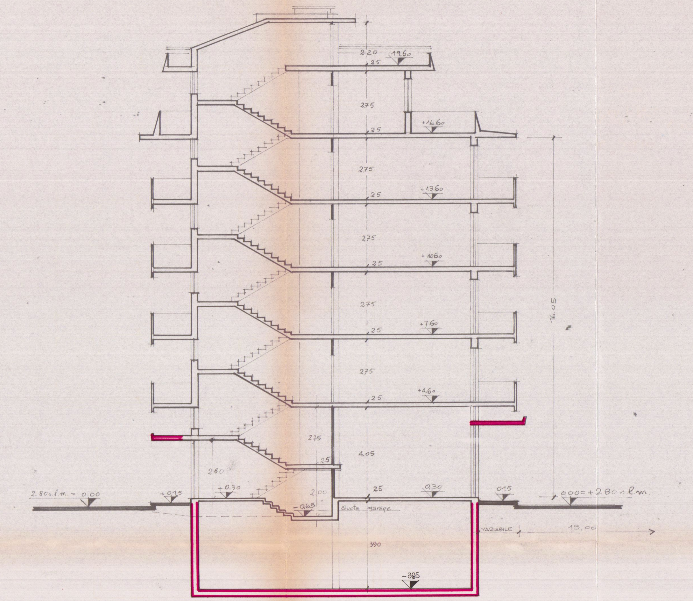
SEZIONE TRASVERSALE
